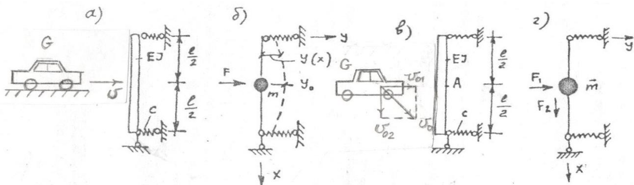
Рисунок 3 – Расчетные схемы балки барьеры безопасности на упругих опорах а-схема упругоопертой балки на лобовой удар; б-динамическая расчетная схема; в-то же на касательной удар и соответствующая расчетная схема
