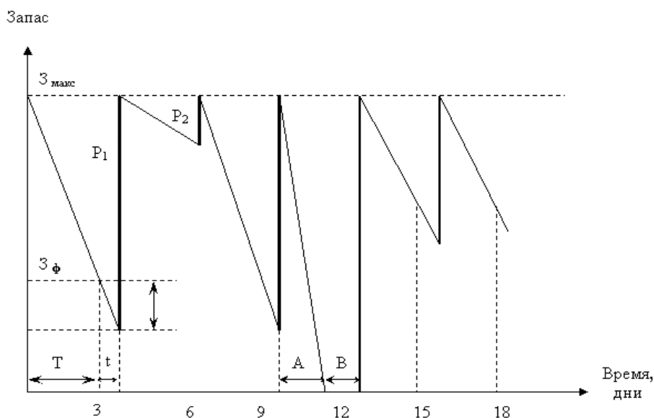
Рисунок 1 - Система контроля за состоянием запасов с фиксированной периодичностью заказа
