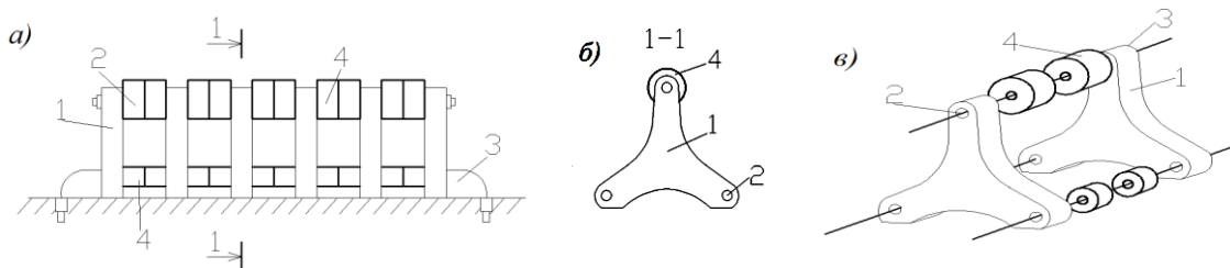
Рисунок 1 – Разделитель полос встречных движений смешанного типа а) фасад; б) разрез по 1-1; в) схема сборки – для иллюстрации элементы расположены в растяжку; 1-триада; 2-отверстие; 3-трос; 4-резиновые прокладка
